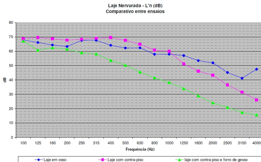
Figura 1 – Comparativo entre os Níveis de Ruído de Impacto Normalizados (L'n).
